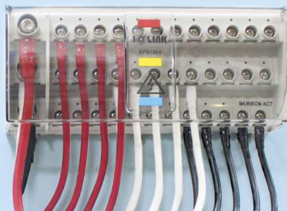
BPS シリーズ 配線型ブスタータイプの 電源分配ブロック
